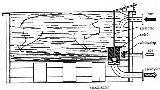
33. ábra. Úsztatásos forrázókád
