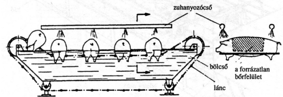
34. ábra. Bölcös forrázókád
