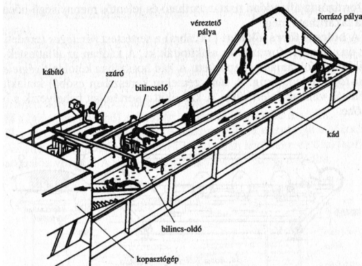
35. ábra. Vonszolásos forrázókád
