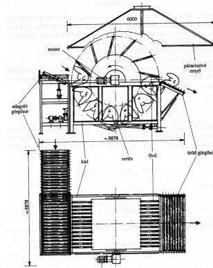
36. ábra. Forgó forrázókád
